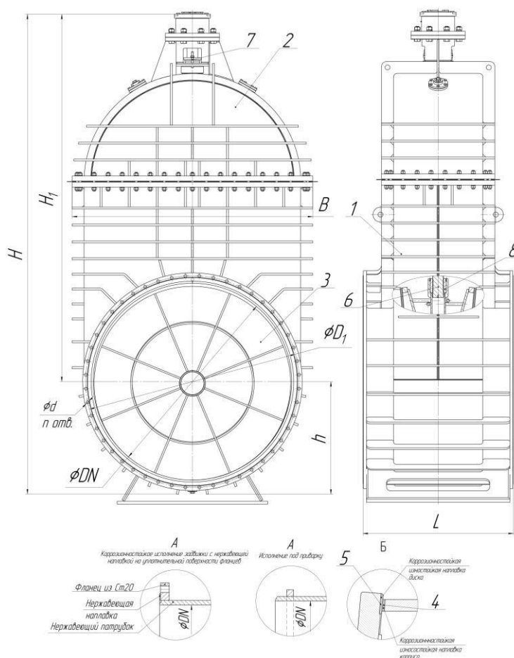
Габаритный чертеж
